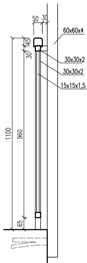
REZ a-a' M 1:25
