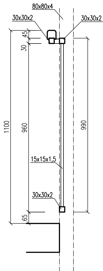
REZ b-b' M 1:25
